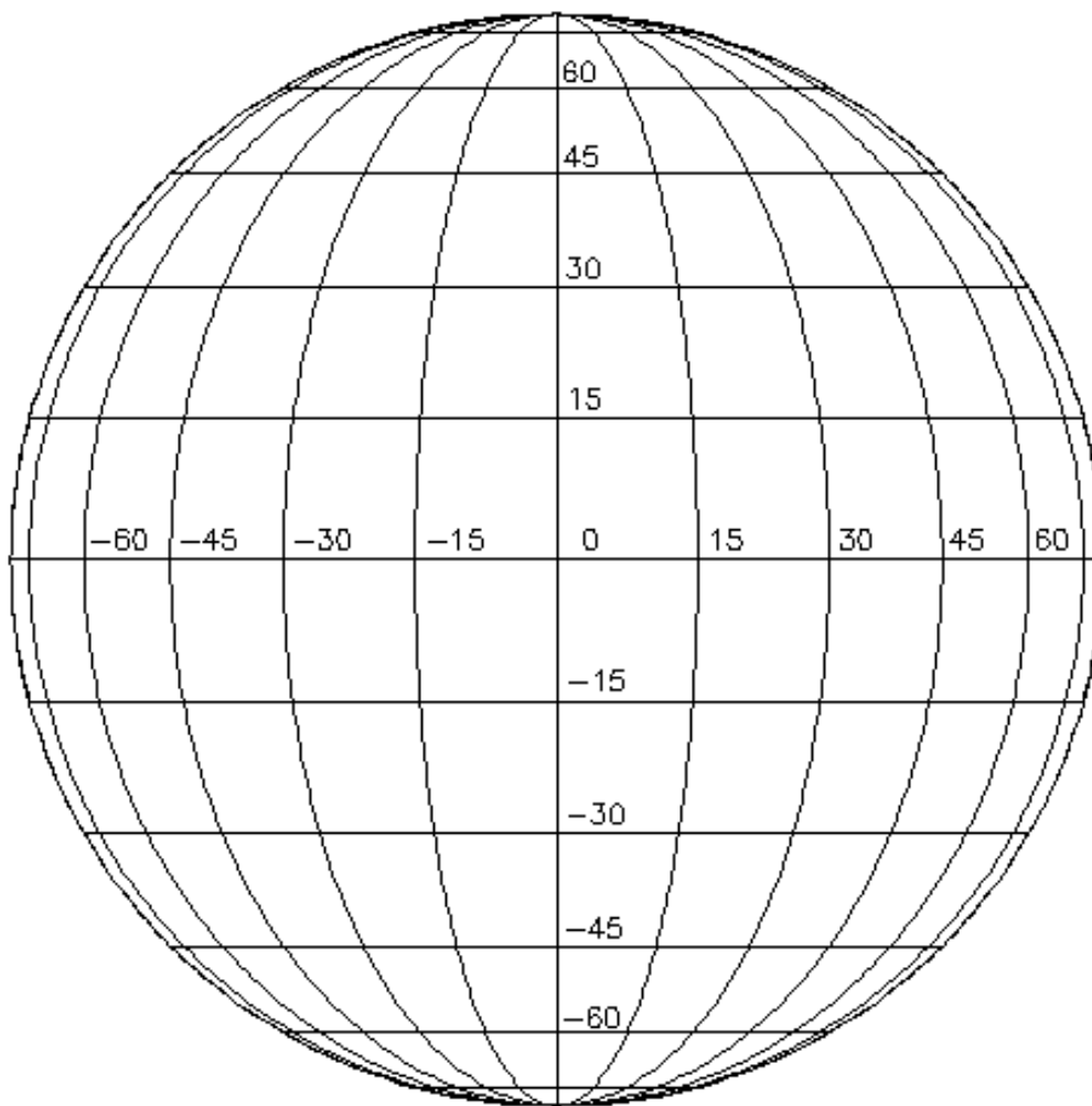
Solar Coordinates B=+0
